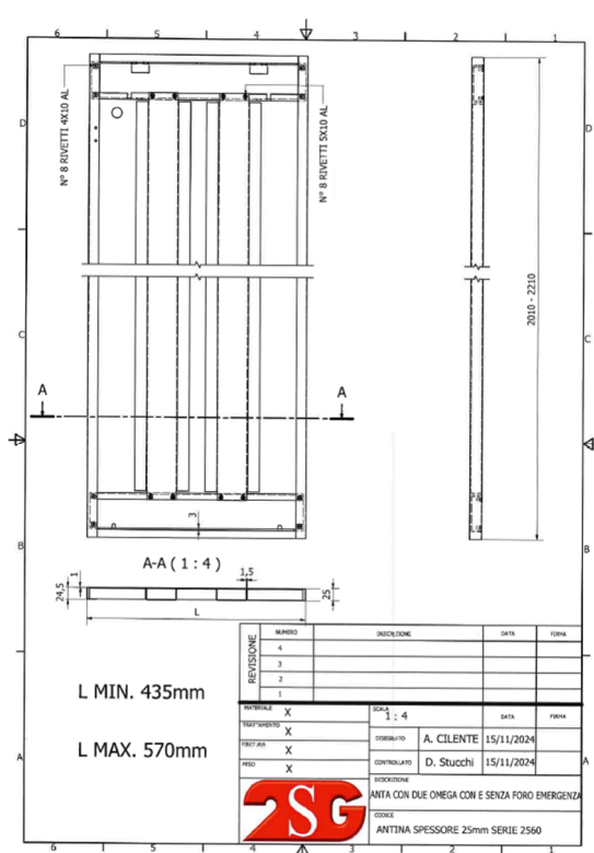
Anta Serie 2560 con due omega Larg. 435-570mm
