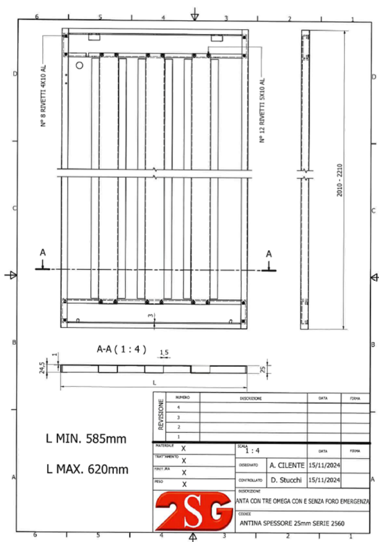
Anta Serie 2560 con tre omega Larg. 585-620mm
