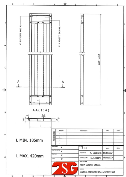
Anta Serie 2560 con un omega Larg. 185-420mm
