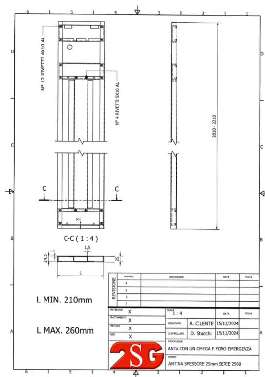
Anta Serie 2560 con un omega Larg. 210-260mm
